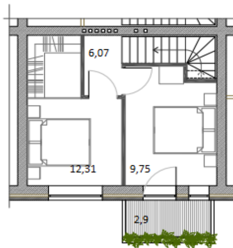
План 2 этажа
