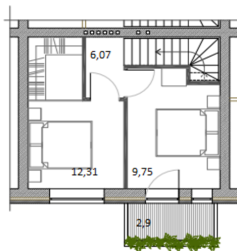
План 2 этажа
