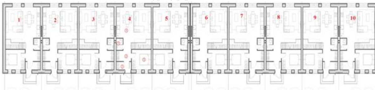
План 2 этажа
