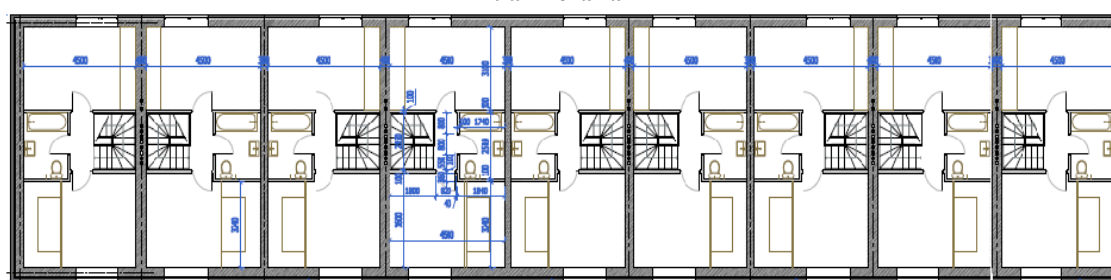
План 2 этажа
