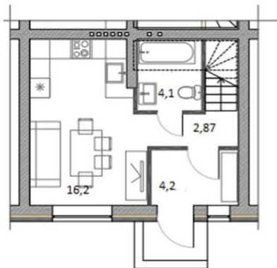
План 1 этажа
