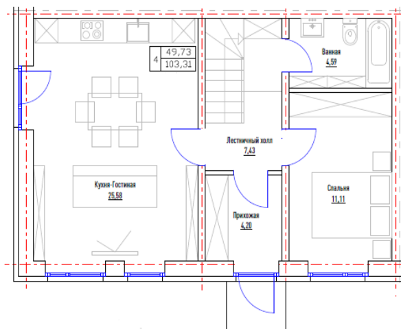
План 1 этажа
