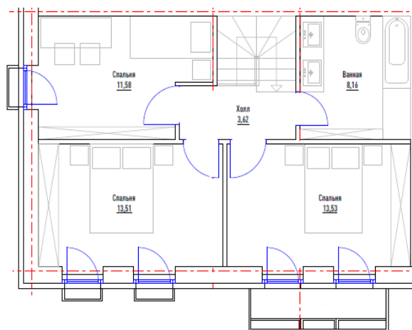
План 2 этажа
