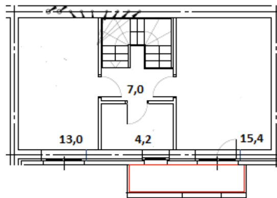
План 2 этажа
