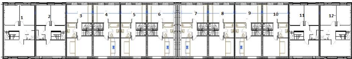
План 2 этажа
