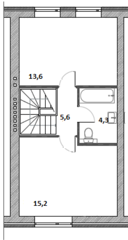
2 этаж
