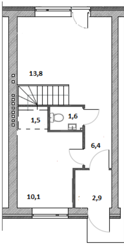
1 этаж
