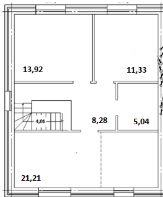
2 этаж
