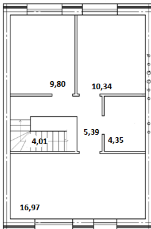
2 этаж
