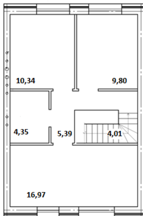
2 этаж
